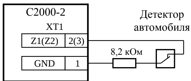
Рисунок 15 Схема подключения детектора автомобиля с "нормально-замкнутыми" контактами в ШС1 и ШС2 контроллера "C2000-2"
