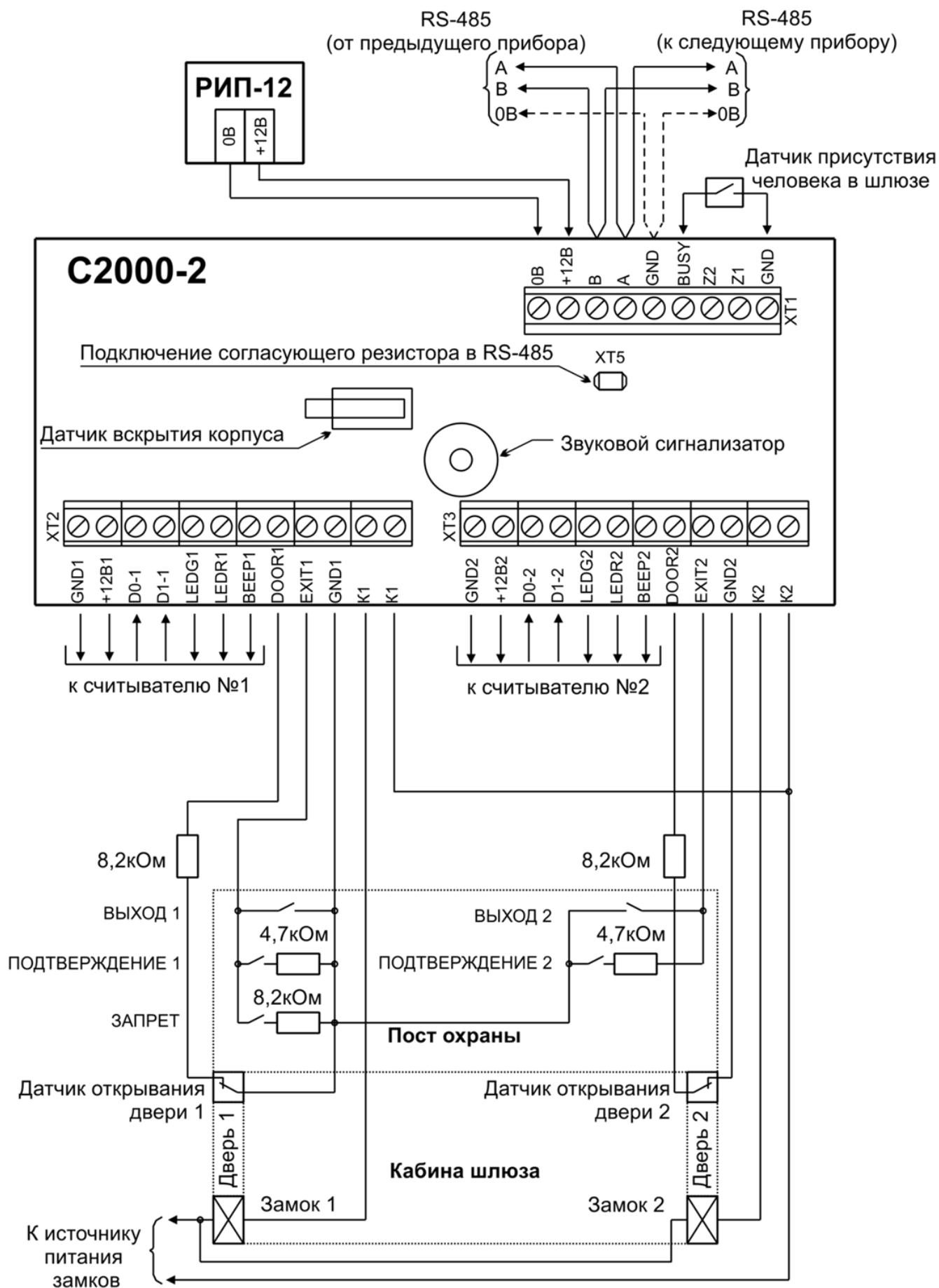
Рисунок 16 Схема подключения контроллера "C2000-2" в режиме "Шлюз"
